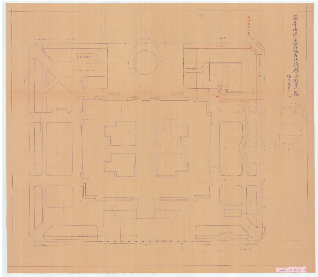
圖 3-11：高等法院及台北地方法院廳舍配置圖
